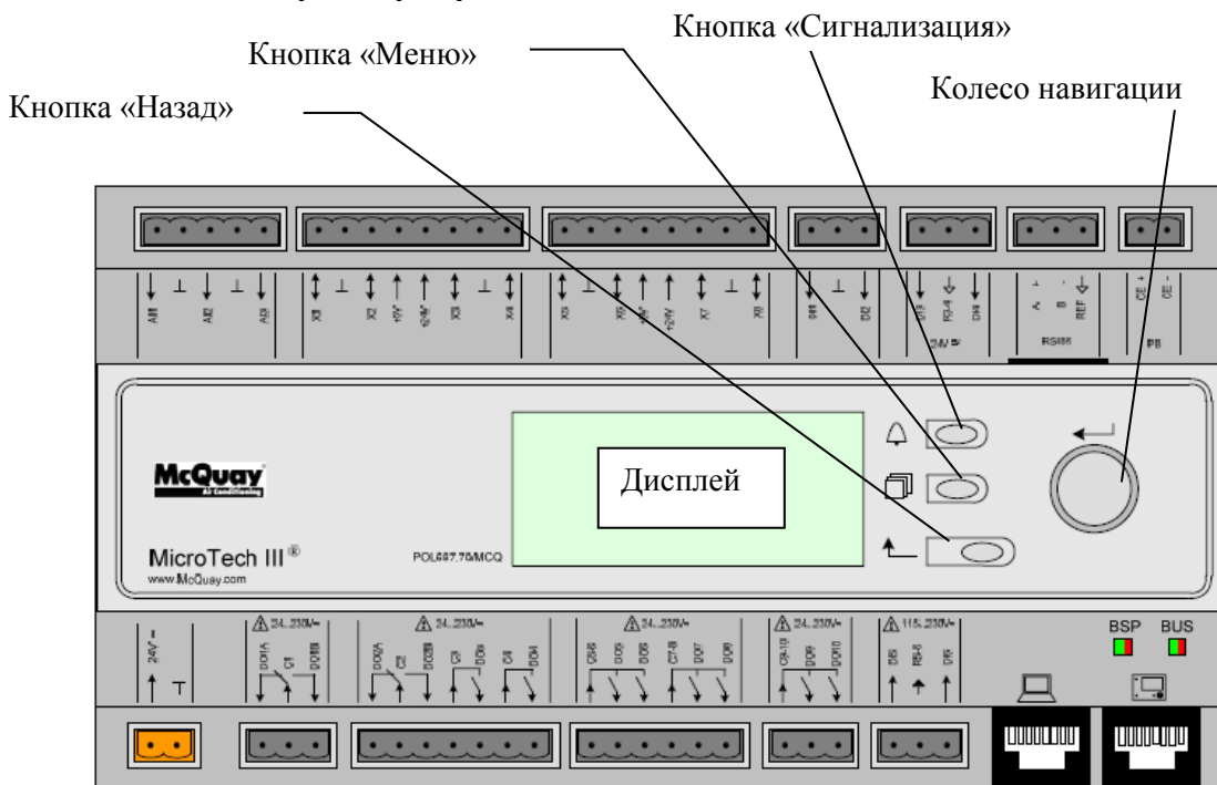
Рис. 7. Контроллер агрегата
