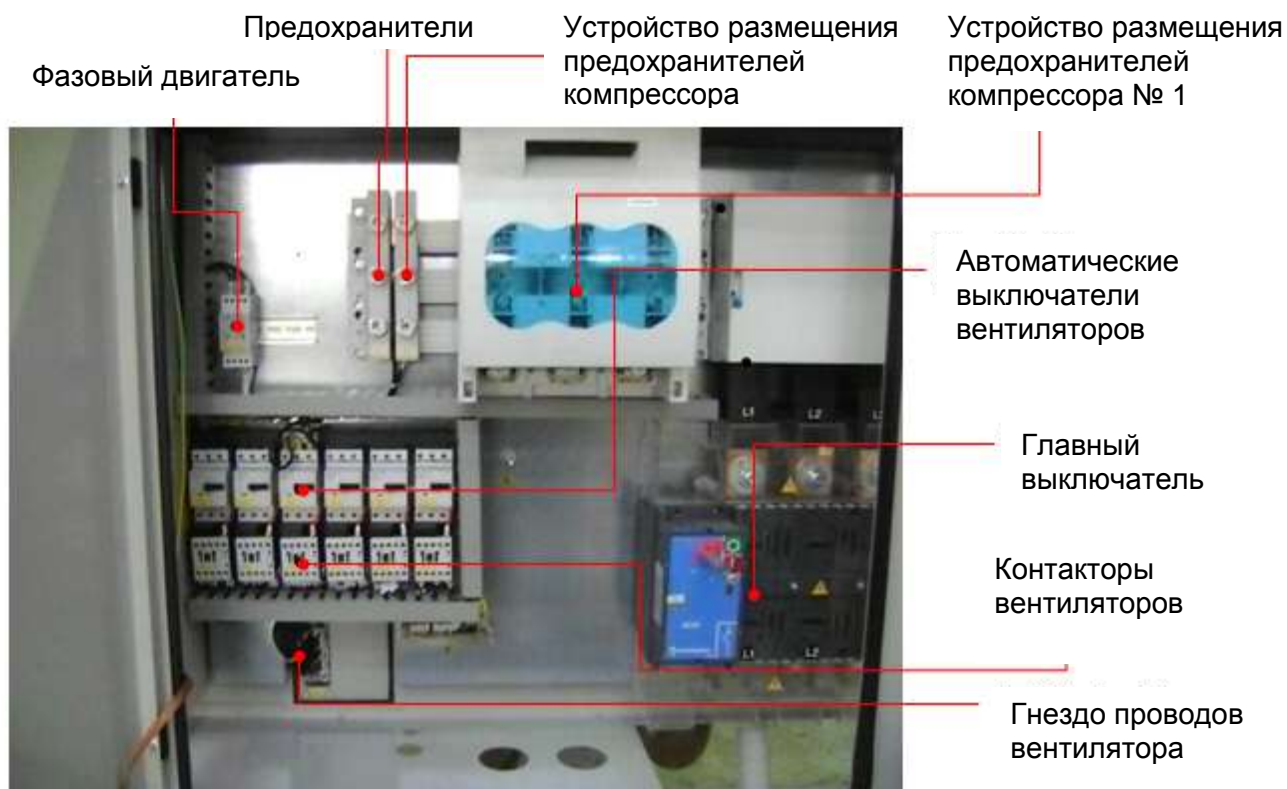
Рис. 2. Силовая панель, левая сторона
