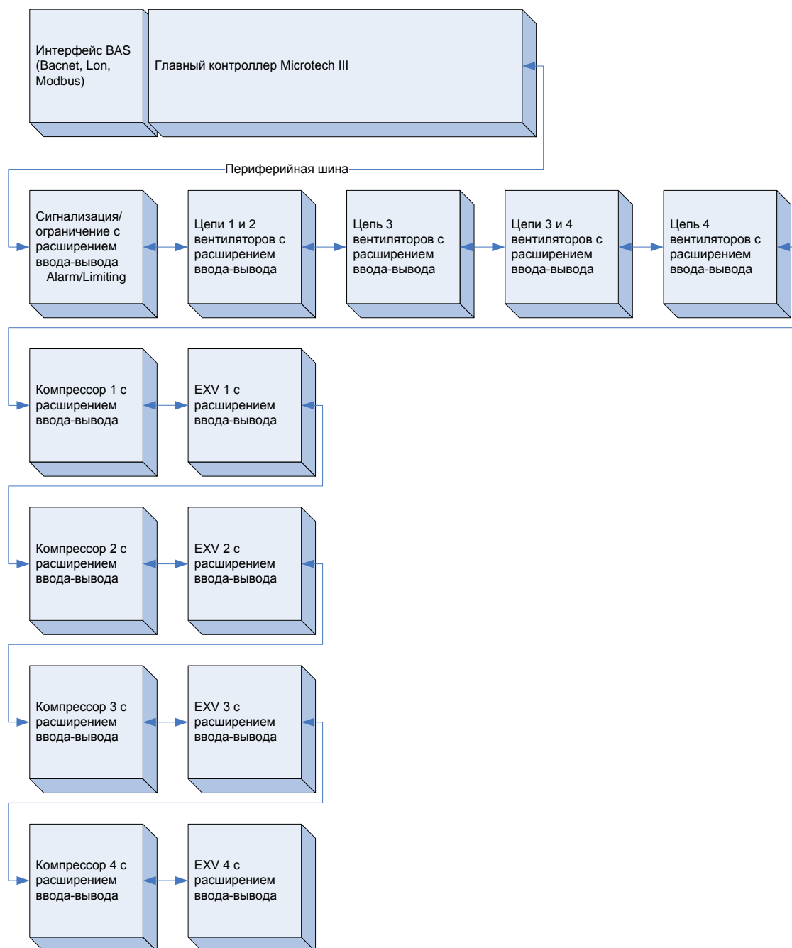
Рис. 4. Архитектура системы
