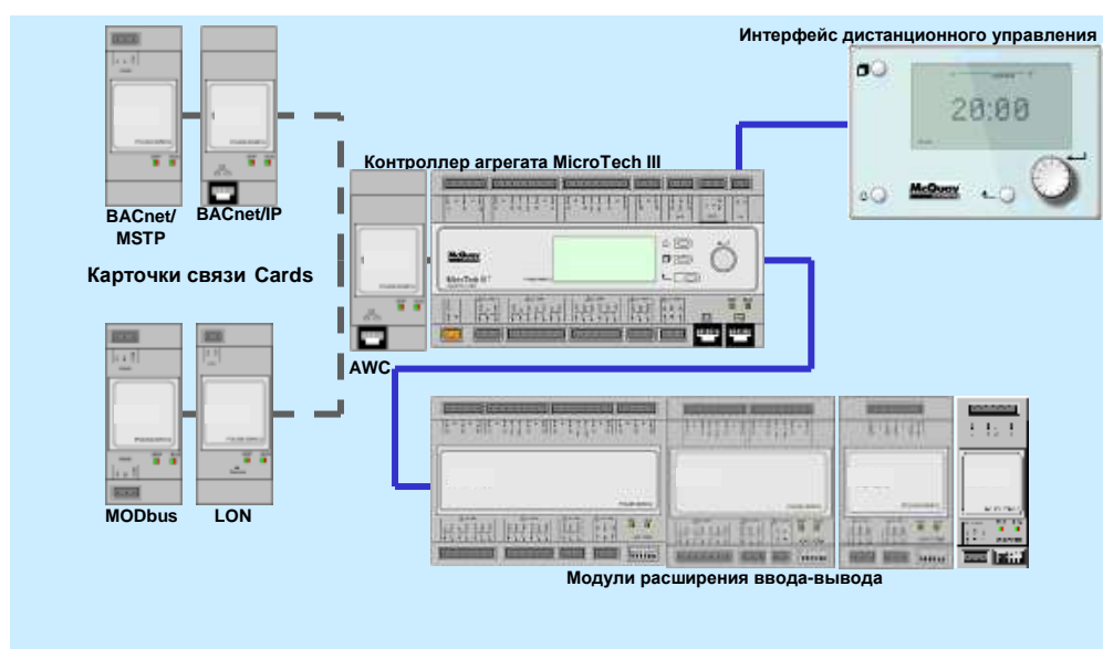
Рис. 6. Аппаратная структура
