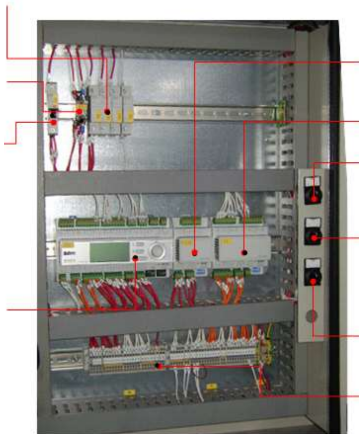
Рис. 1. Элементы панели управления
