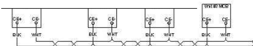
Подключение цепочкой до 8 агрегатов к одному удаленному интерфейсу
