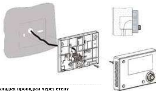
Прокладка проводки через стену
